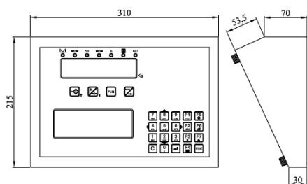
Detall tècnic
