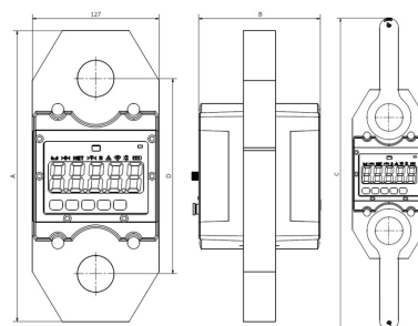
Detalle técnico
