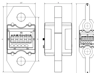
Detall tècnic
