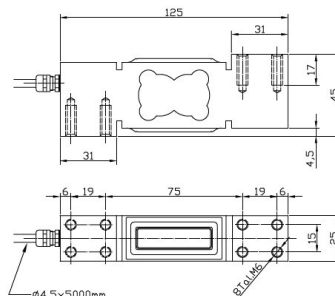
Plànol acotat de la PL-50; cotes en mil·límetres i cable de 5000 mm.
