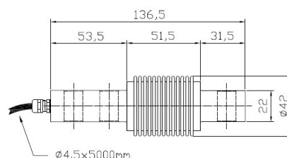
Plànol tècnic de la FX-2.
